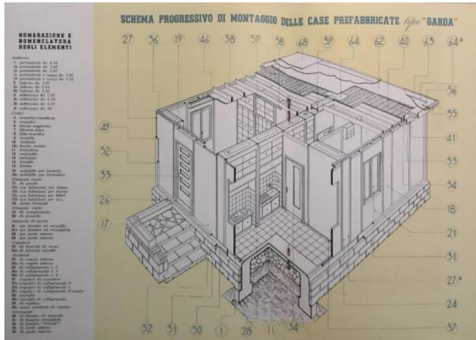
Casa prefabbricata Garda di Legnami Pasotti (Catalogo S.A. Legnami Pasotti, Case prefabbricate tipo Garda)
