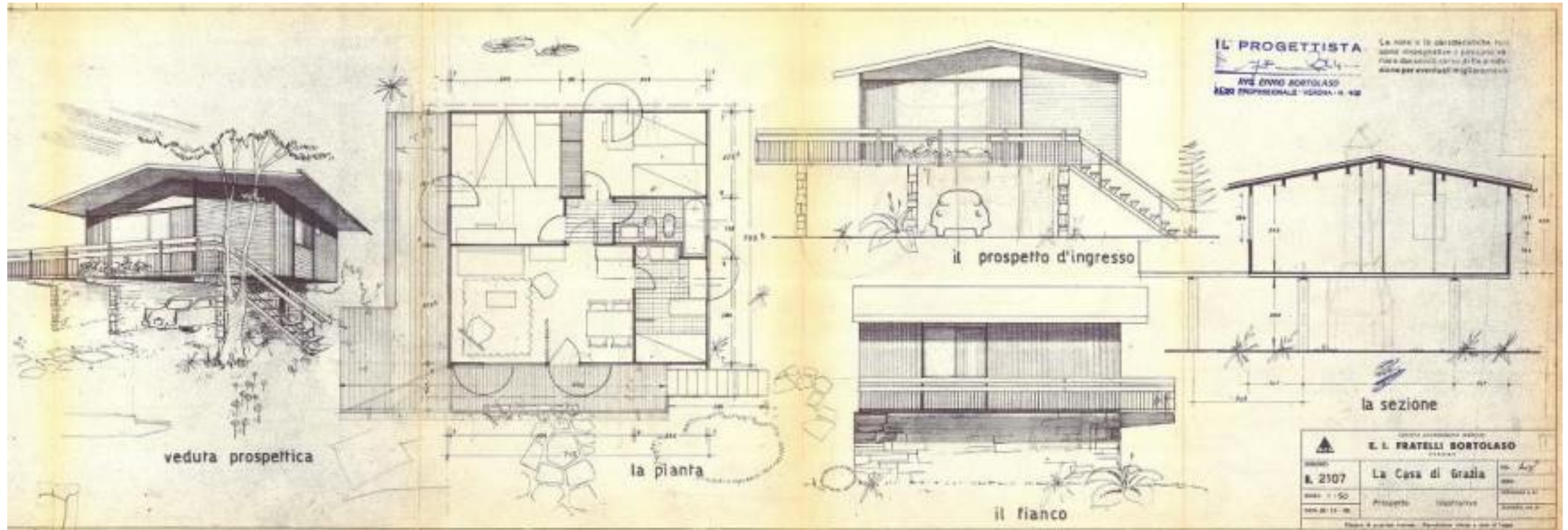
Elaborati di progetto della casa di "Grazia", Fratelli Bortolaso, 1958 (Archivio Piero Bottoni, DASTU-Politecnico di Milano)
