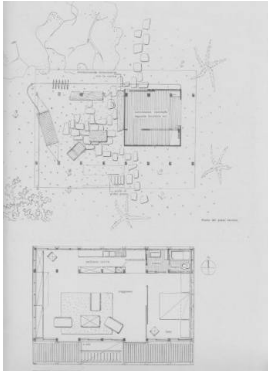
Vittorio Gandolfi, Luigi Tanzi. Casa in legno smontabile, 1944 ("Domus", 203, 1944)
