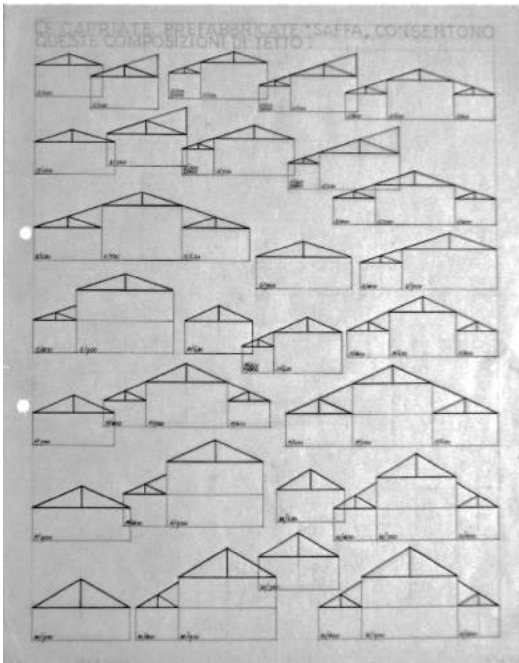
Gio Ponti. Progetto di casetta con tetto a falde su capriate prefabbricate Saffa, 1944-45 (CSAC-PON; Courtesy Gio Ponti Archives)
