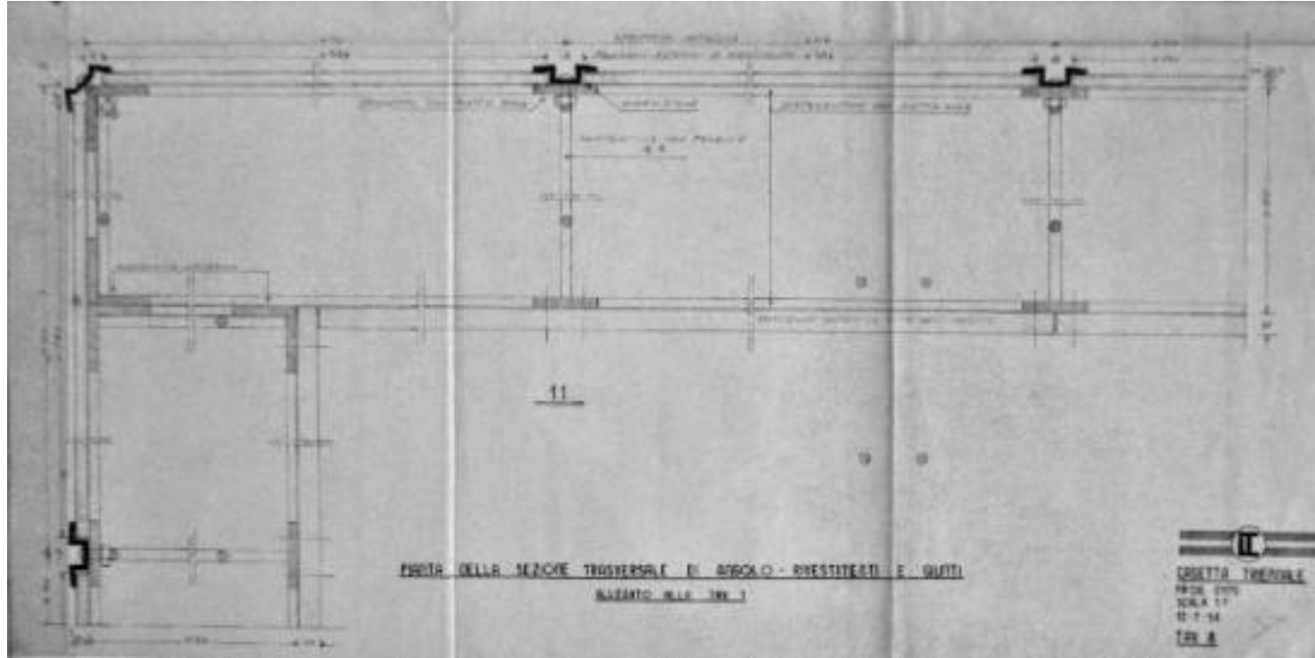
Ponti, Rosselli, Fornaroli. Casa unifamiliare di serie, X Triennale, 1954 (CSAC-PON; Courtesy Gio Ponti Archives)
