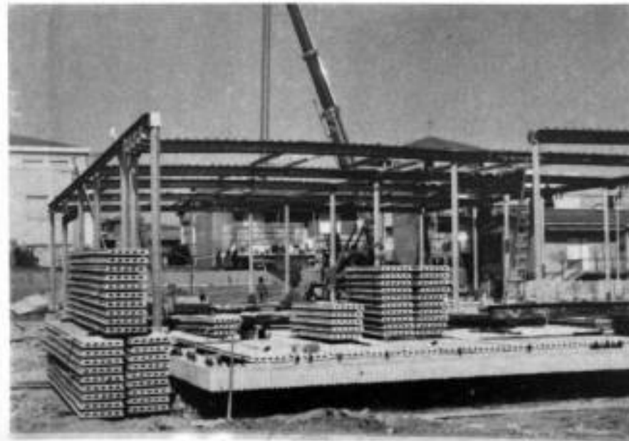
Montaggio di pilastri e travi metalliche e pannelli in C.A.P. cemento armato prefabbricato. Il cantiere si presenta in forma diversa rispetto alla struttura in cemento armato. Si ha la sensazione di un edificio frutto di lavoro industriale fuori opera.
