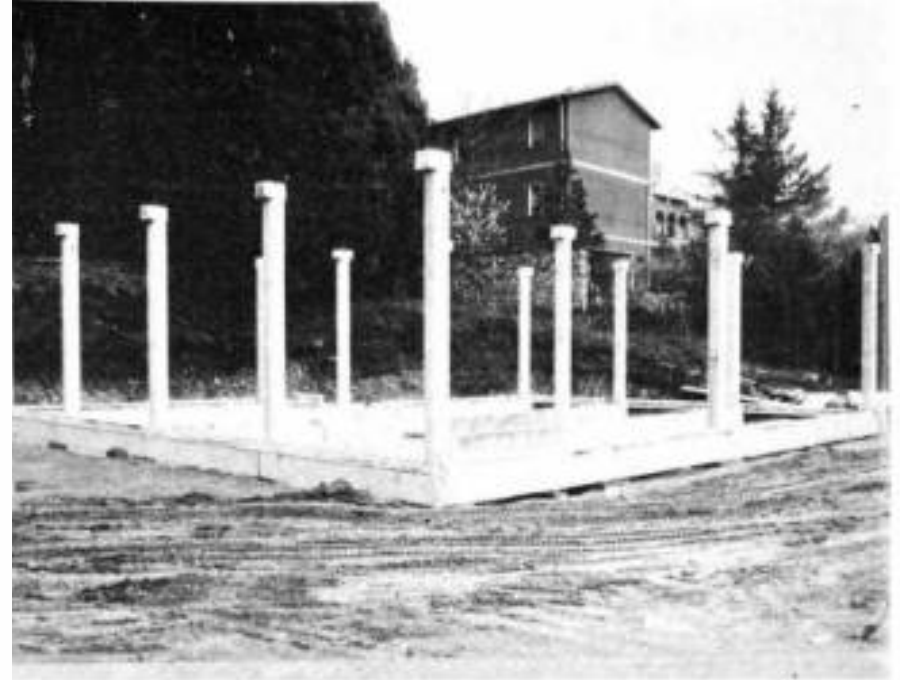
Struttura di questo edificio è in pilastri e travi di cemento armato prefabbricate, trasportate e montate in opera su fondazioni continue precostituite.
