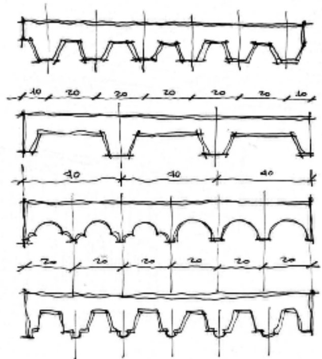
Studi di profili per le pannellature esterne
